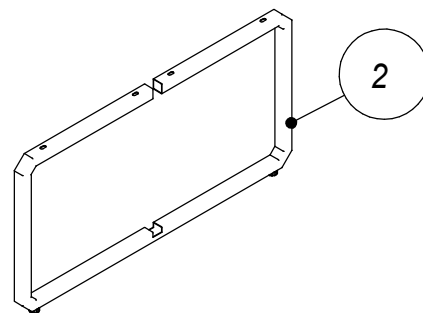
Опора стола нижняя - 1 шт. (с присадкой для колесных опор)
